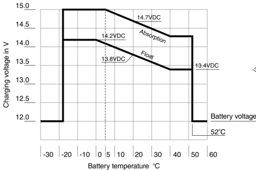
Schéma 10. Compensation en température sur les modèles CX12xx
